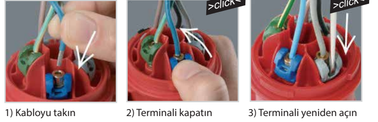
1) Kabloyu takın
