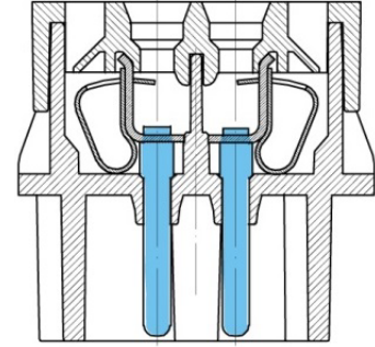
Yaylı Bağlantı
